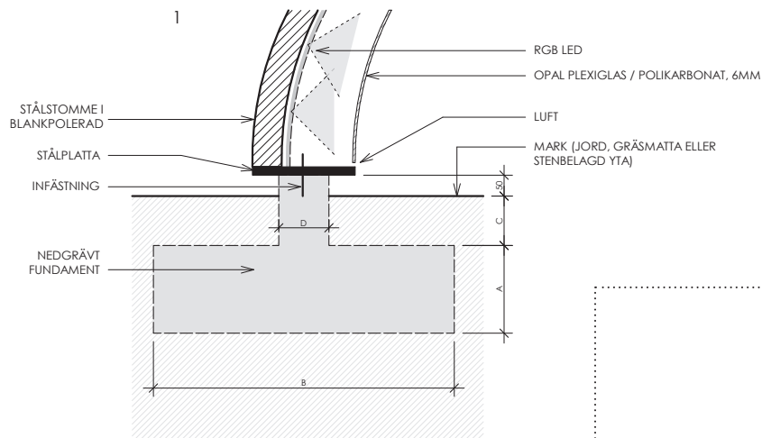
1. Detalj på fundament. 2. Detalj på stålstomme.
