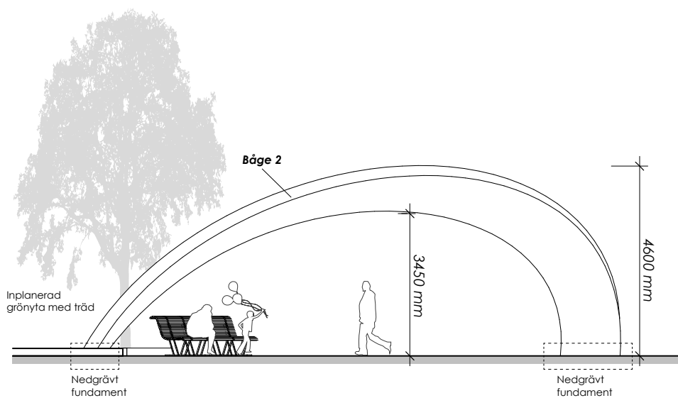
Elevation Båge 2
